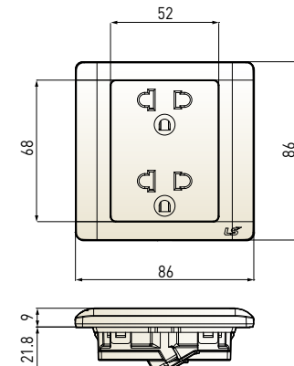
Double 3Pole socket
